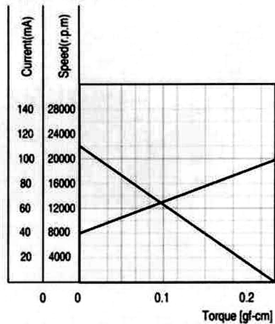
特性图 Characteristics
