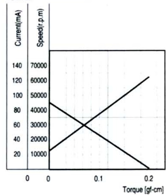
特性图 Characteristics
